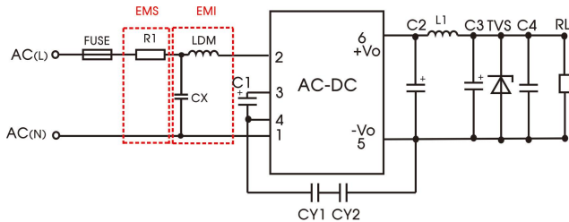
推荐电路 2
