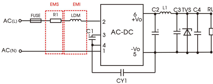
推荐电路 1
