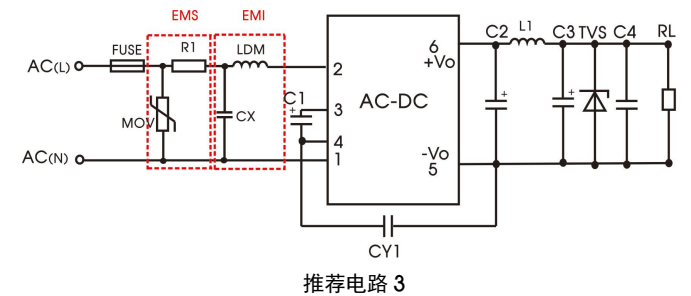
推荐电路 3
