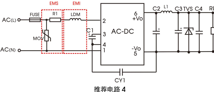
推荐电路 4
