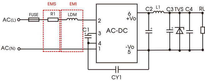
推荐电路 1
